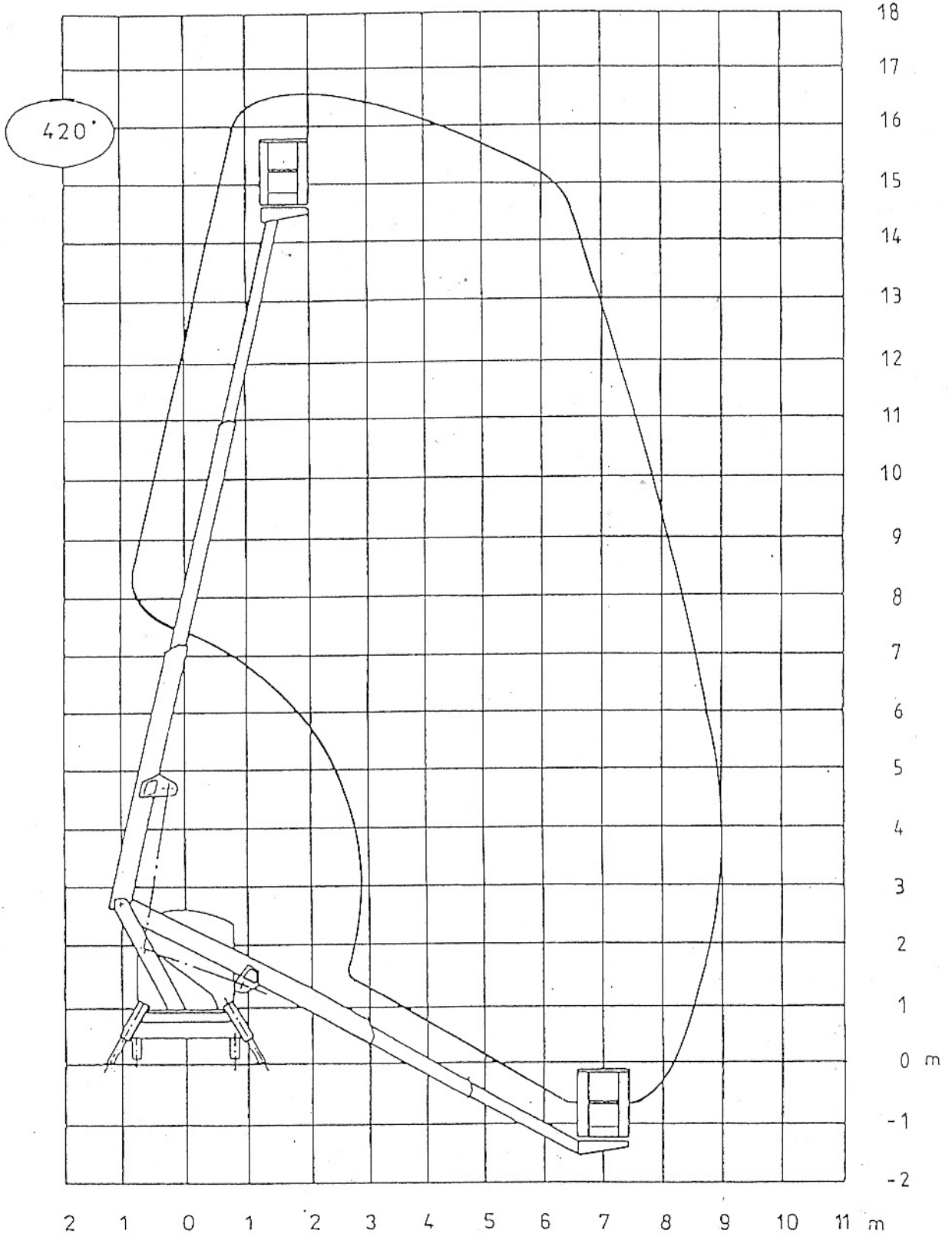
Arbeitsbereich WT 165
